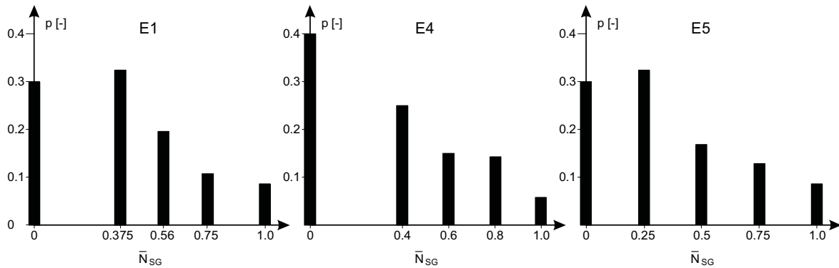
Rys. 6. Histogramy rozkładu obciążeń silników pracujących przy cyklach prób: E1, E4 i E5 [4-6] Fig. 6. Histograms of distribution of engine loads upon tests: E1, E4 i E5 [4-6]
