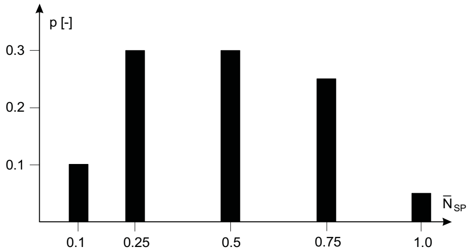
Rys. 5 Histogram rozkładu obciążeń silników pomocniczych pracujących przy n_{SP} = idem [4-6] Fig. 5 Histogram of distribution of auxiliary engine loads upon n_{SP} = idem [4-6]
